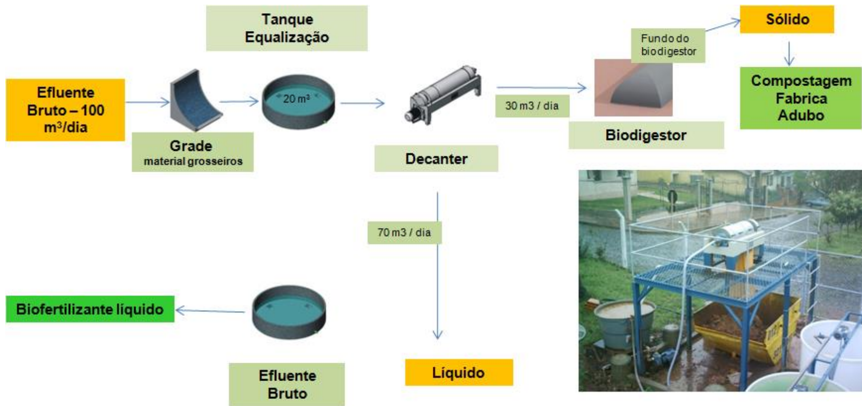
Figura 4: Representação esquemática de um sistema de separação de sólidos + Biodigestor de alta taxa + compostagem.
