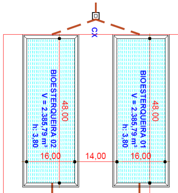
Figura 2: Exemplo esquemático de sistema de esterqueira ou lagoas.
