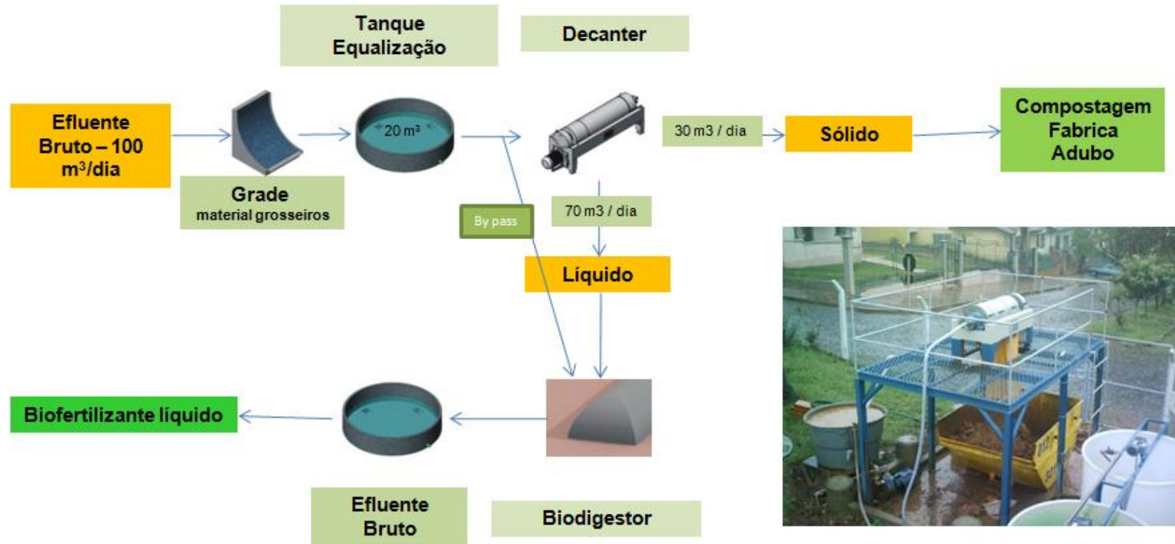
Figura 3: Representação esquemática de um sistema de separação de sólidos e compostagem.
