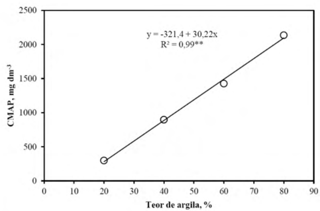
Figura 4. Aumento da capacidade máxima de adsorção de P (CMAP) em função do teor de argila do solo.** significativo ao nível de 1% de probabilidade de erro.
